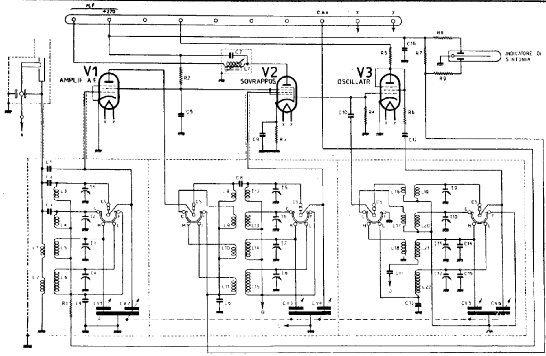
— PHONOLA (S. A. FIMI). — Mod. 617. — Complesso A. F. — Serie ultraconverto. — Produzione 1938-39. — Media frequenza: 470 kHz.
